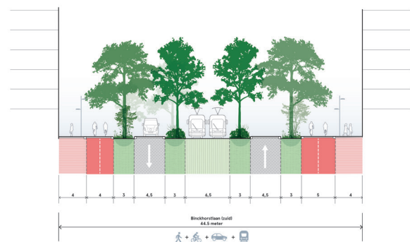
Indicatieve profielen Binckhorstlaan noord, midden en zuid
