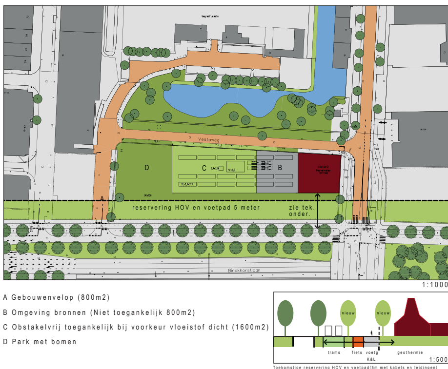
Afbeelding 1-1 Schematisch ruimtebeslag Geothermiecentrale aan de Vestaweg in uitvoeringsfase.
